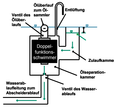
Ölseparationsmodul
